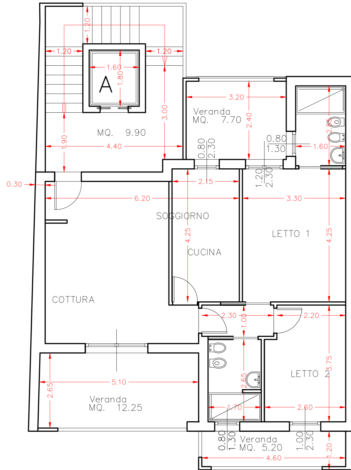
PIANTA P. 2° TRIVANO CUCINA ABITABILE
