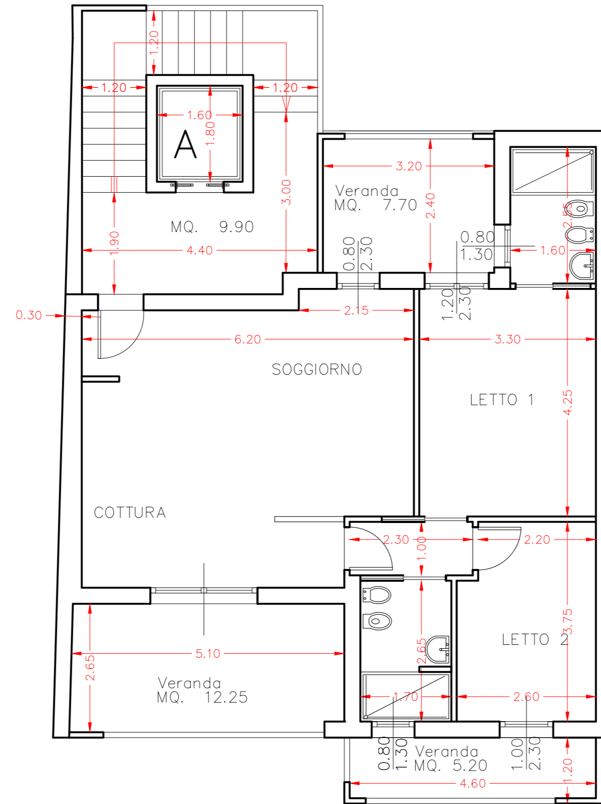
PIANTA P. 2° TRIVANO OPEN SPACE
