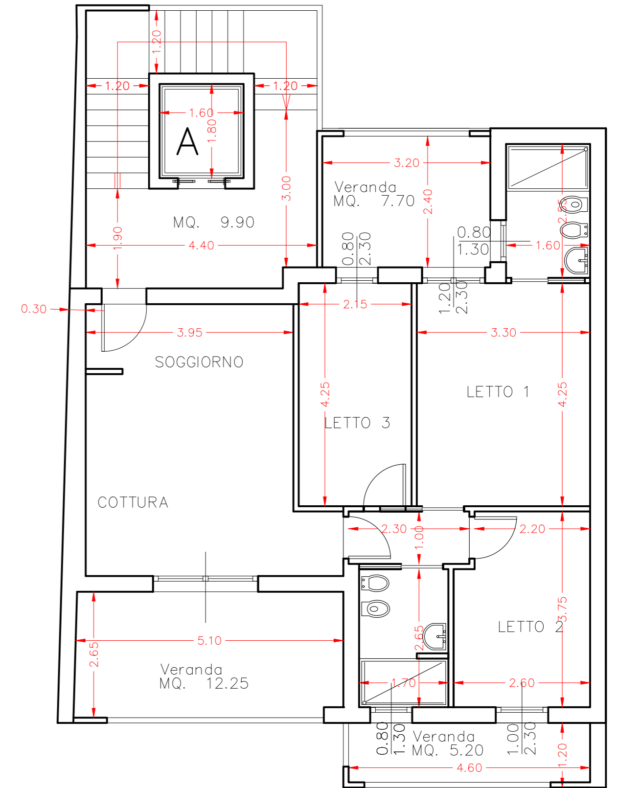
PIANTA P. 2° QUADRIVANO ANGOLO COTTURA
